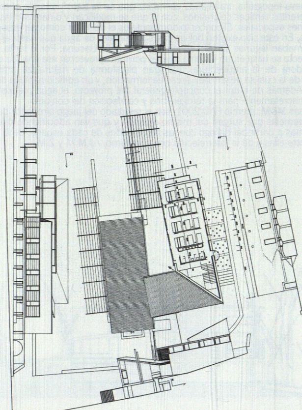
29 · PLANTA ALTA Y ALZADOS
